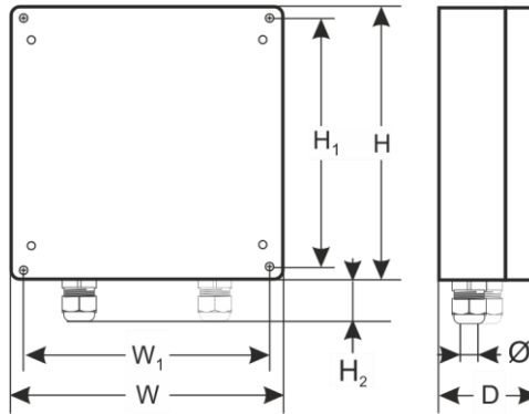
Rys.2. Widok zasilacza.
