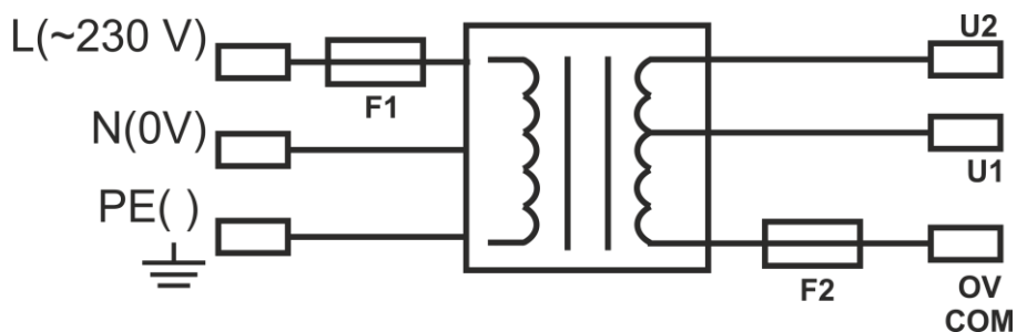
Rys.1. Schemat blokowy zasilacza.
